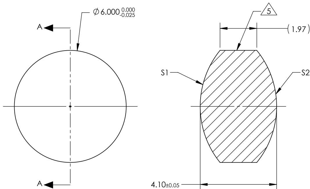
SECTION A-A
