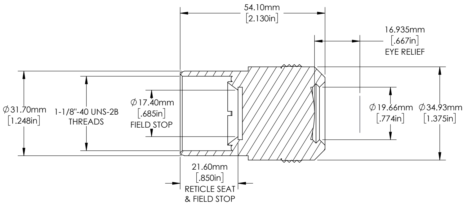
SECTION A-A
